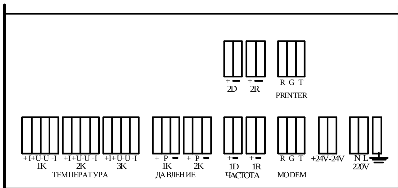
Рис. 5. Блок ИВУ
