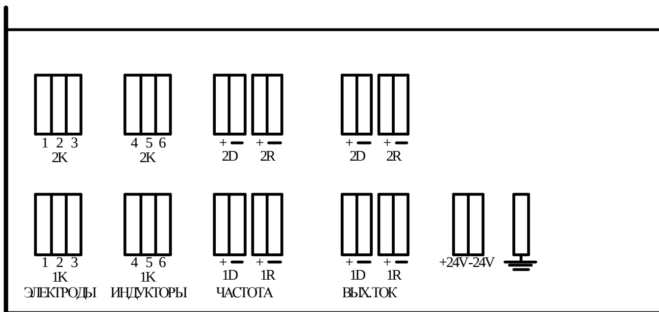
Рис. 4. Блок ПНЧ
